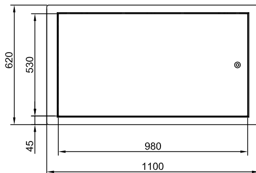
Boven aanzicht
